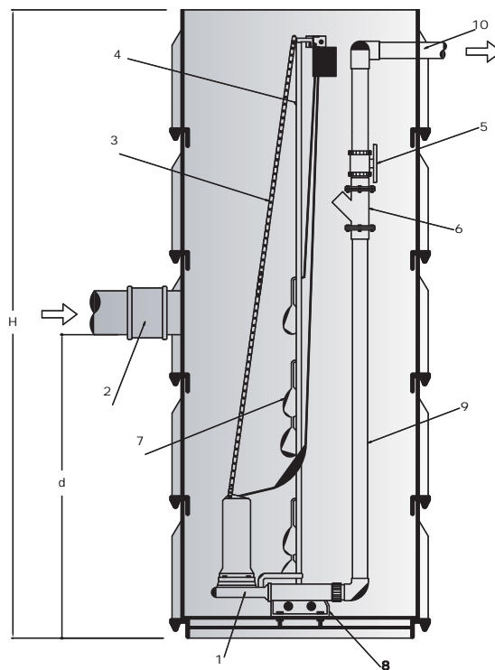
alzado
