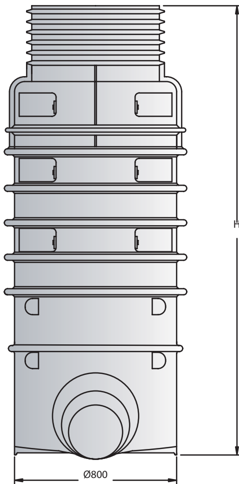
perfil
