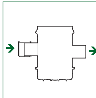
arqueta Ø400 registrable decantadora
