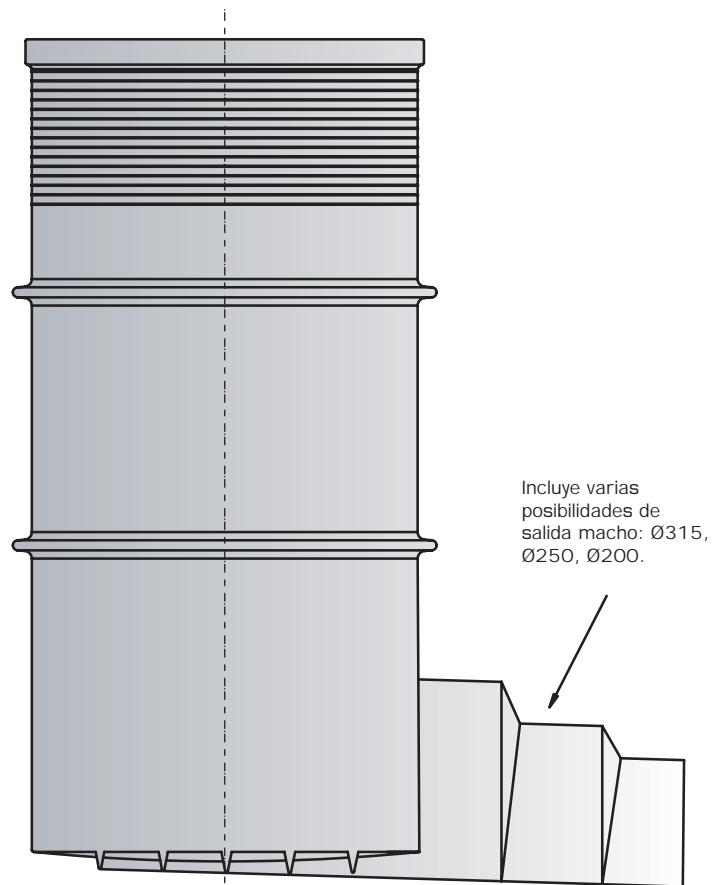
alzado
