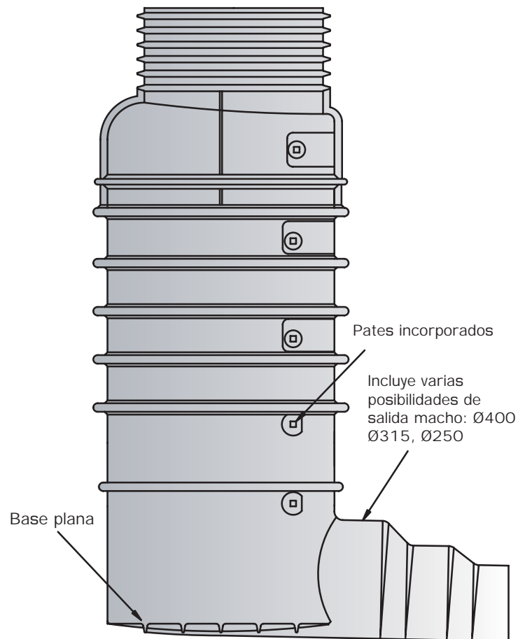
alzado
