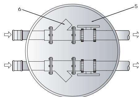
detalle pozo con válvulas
